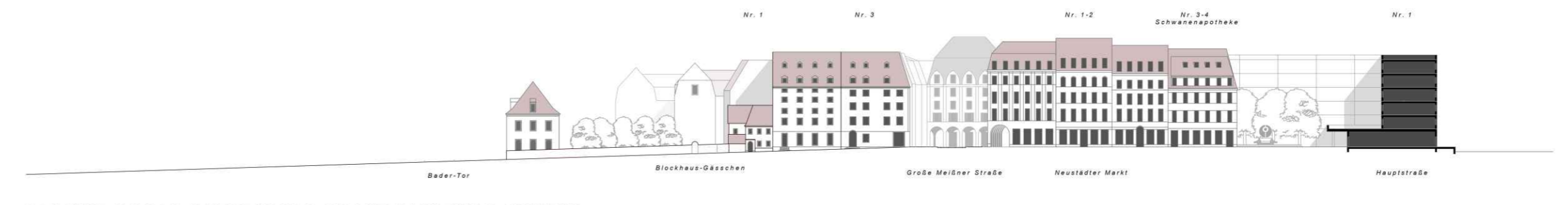
SCHNITT DURCH NEUSTÄDTER MARKT RICHTUNG WESTEN
